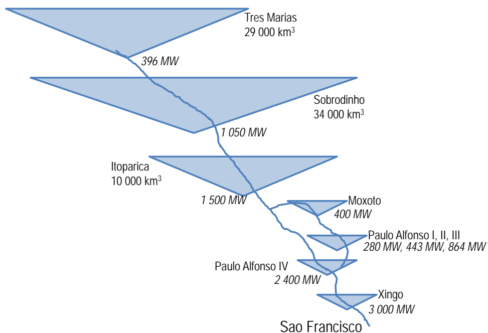
Figure 4.A5.1. As usinas hidrelétricas do São Francisco
