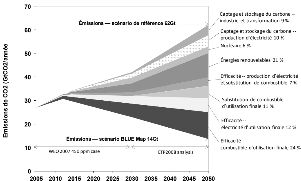
Figure 2. Contribution des principales technologies à l'atténuation du changement climatique Gigatonnes de CO 2 /année, en pourcentage
