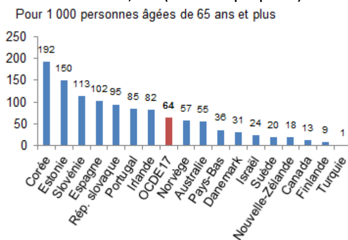
Graphique 6.7. Patients âgés de 65 ans et plus avec prescription de benzodiazépines ou médicaments apparentés à longue durée d'action, 2015 (ou année la plus proche)
