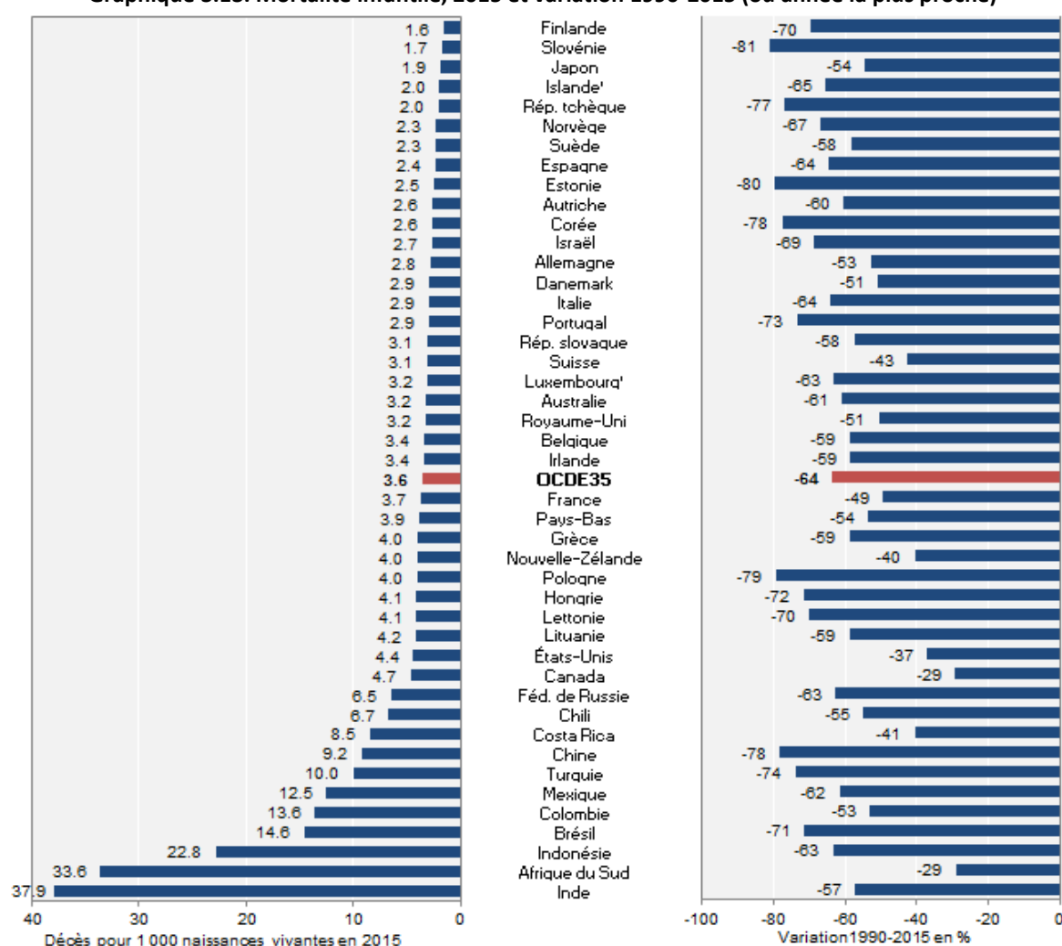
Graphique 3.13. Mortalité infantile, 2015 et variation 1990-2015 (ou année la plus proche)
