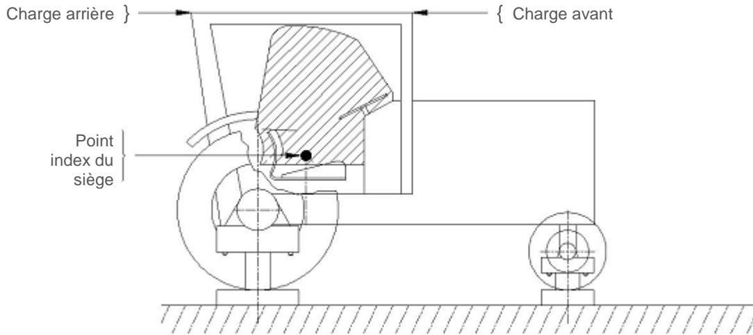
Figure 4.1.a Cabines de protection
