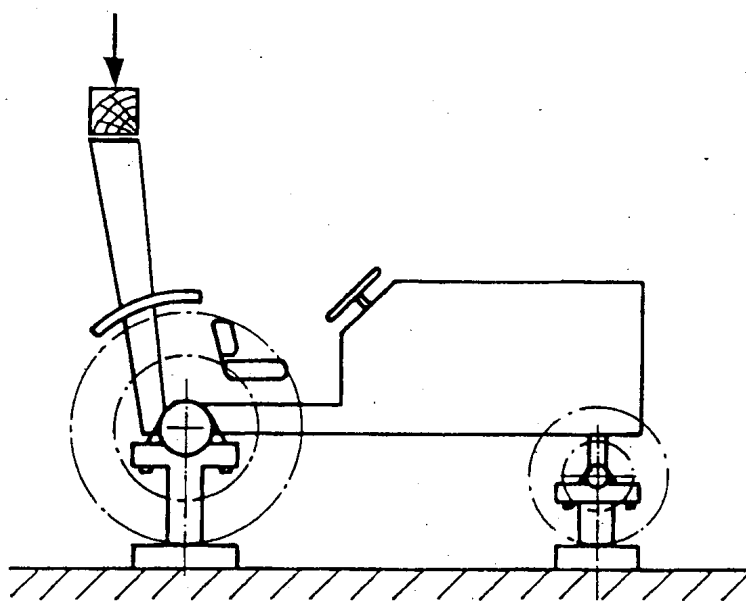
Figure 4.7.b Cadres de protection arrière
