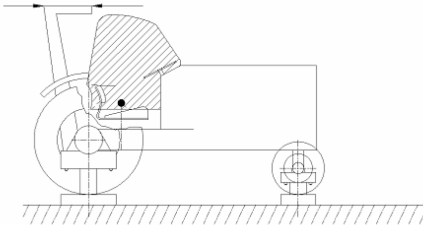
Figure 4.1.b Cadres de protection arrière
