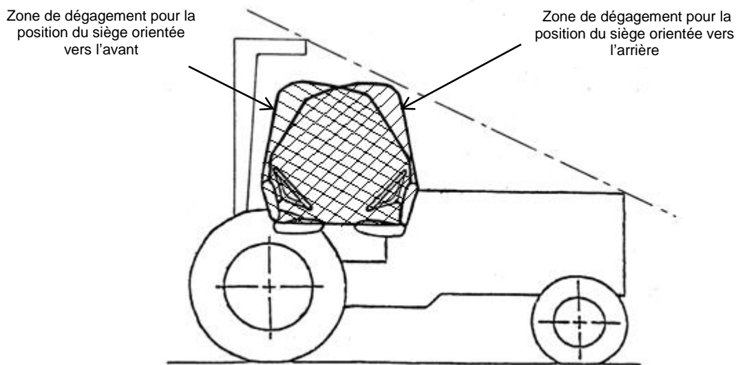
Figure 4.24.b Cadres de protection arrière
