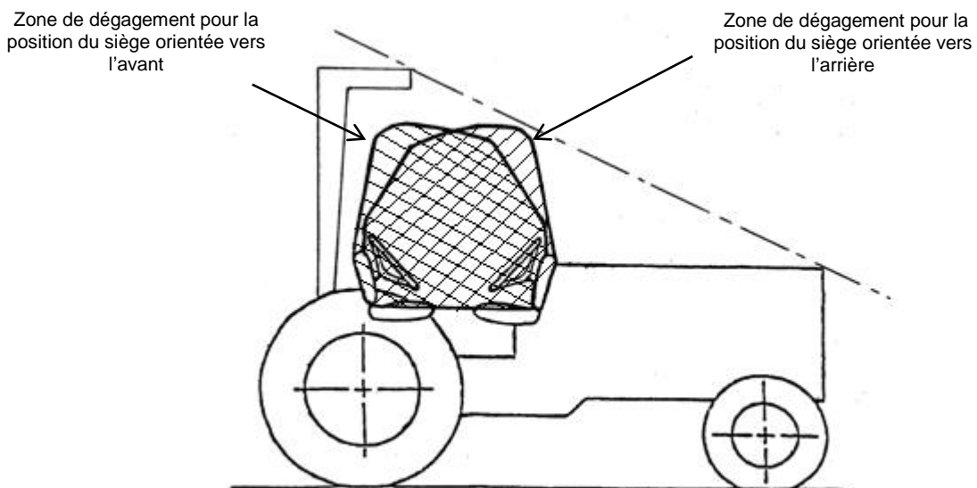
Figure 4.11.b Cadres de protection arrière
