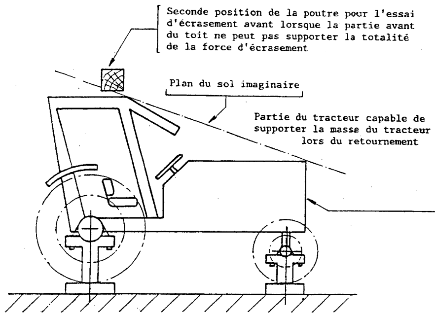
Figure 4.8.a Cabines de protection
