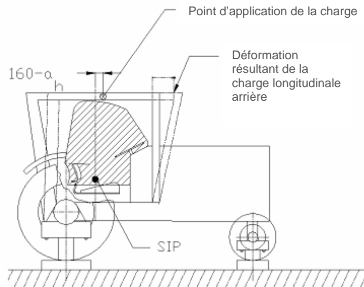
Figure 4.4.a Cabines de protection
