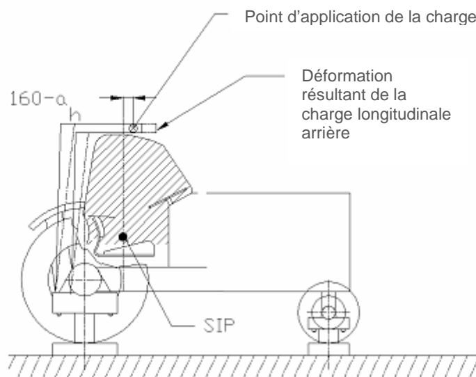
Figure 4.4.b Cadres de protection arrière
