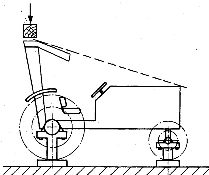
Figure 4.8.b Cadres de protection arrière
