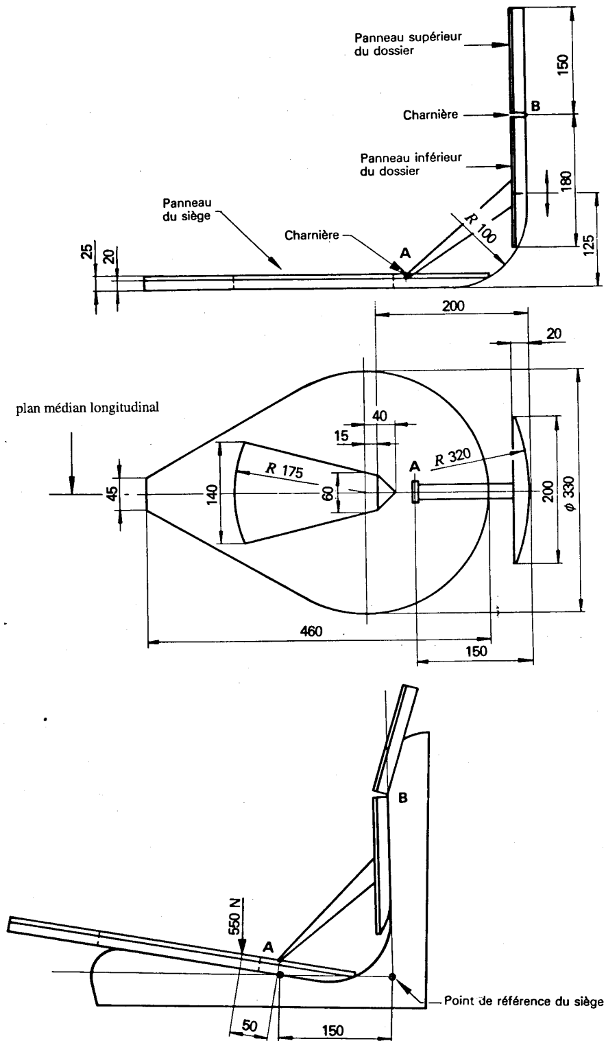
Figures 4.18, 4.19 et 4.20 Dispositif pour la détermination du point de référence du siège
