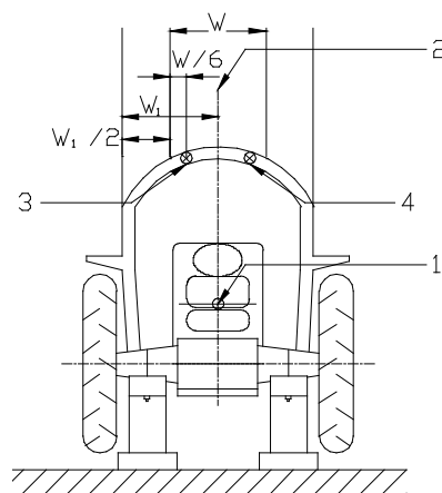
Figure 4.3.a ROPS à 4 montants
